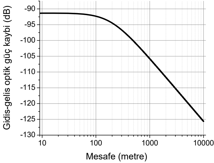
Şekil 12. Eş fazlı algılama için toplam optik kayıp, mesafe ilişik grafiği
