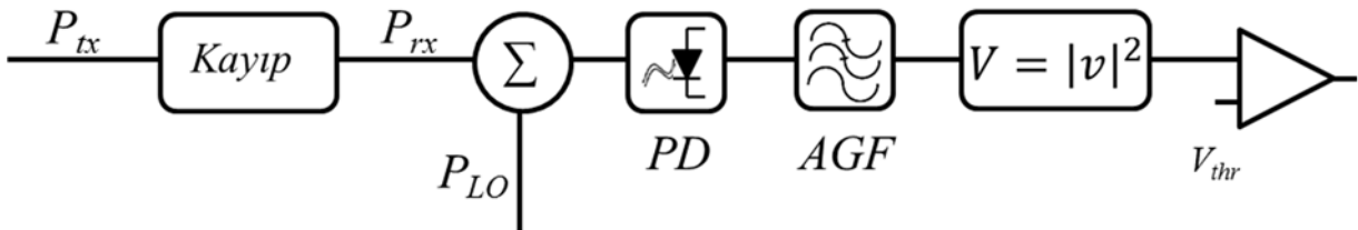
Şekil 13. Tek modlu eş fazlı algılayıcı modeli. AGF: Alçak geçirgen filtre.
