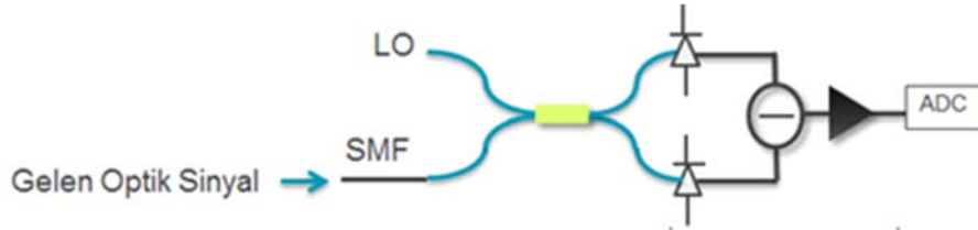
Şekil 6. Tek modlu fiber temelli eş fazlı algılama sistemi
